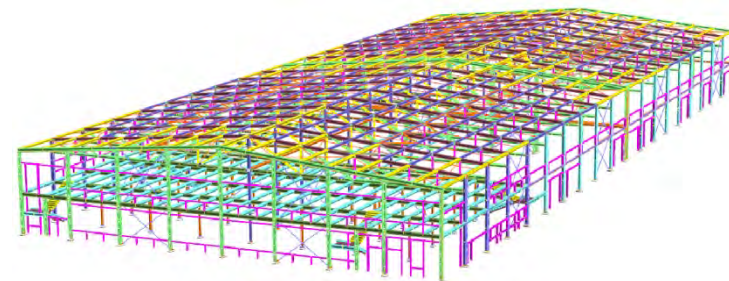
Пространственная схема каркаса
