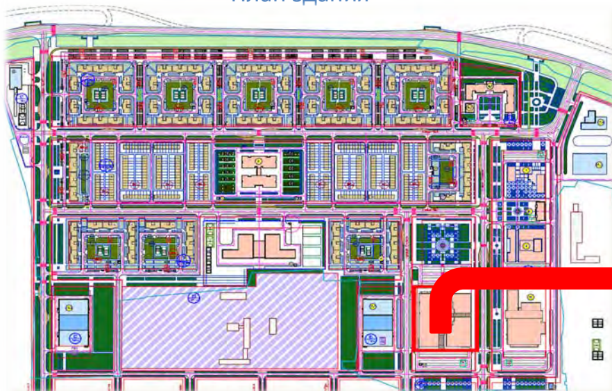
План здания
