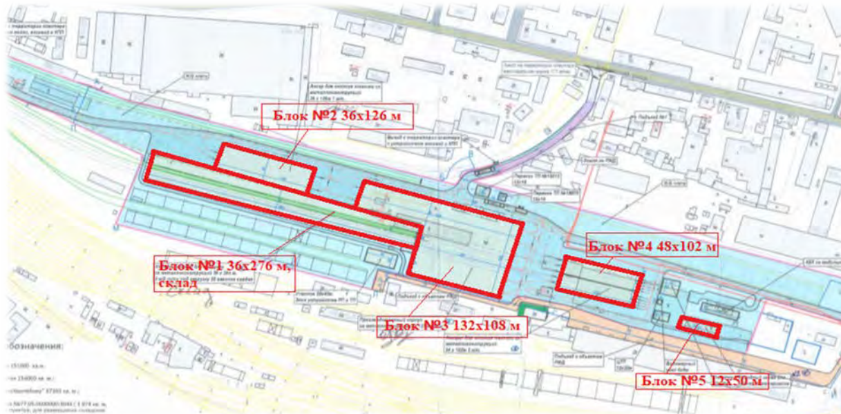
Генплан площадки
